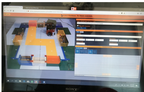
Figura 1. Armazém virtual.
