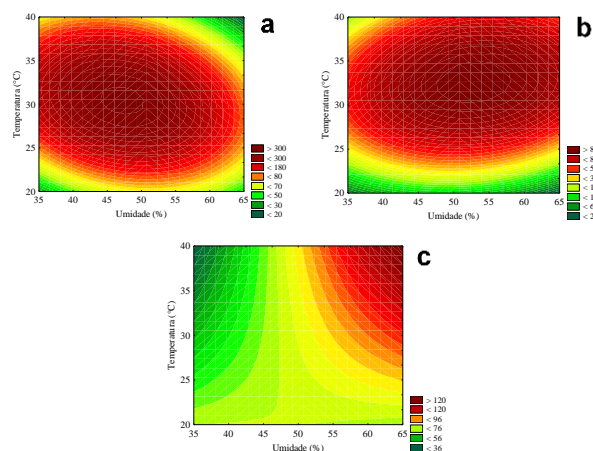
Figura 1. Curvas de contorno para a produção de protease (a) e lipase (b) após 48h de fermentação e fitase (c) após 72h de fermentação semissólida por A. niger LBA02 utilizando farinha de penas de frango como substrato.
