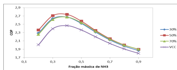
Figura 2: COP em função da fração mássica de NH 3 e das difentes razões de expansão na válvula.
