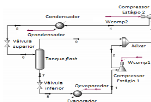
Figura 1: Esquema do ciclo simulado.
