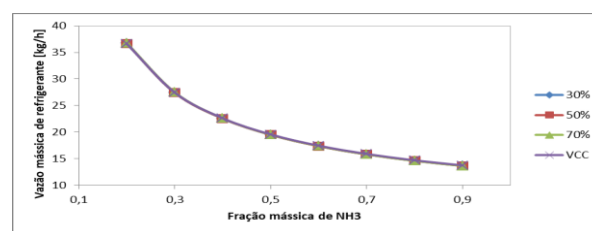
Figura 3: Vazão mássica de refrigerante em função da fração de NH 3 e das razões de expansão na válvula.
