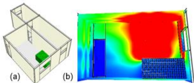
Figura 1. (a) Modelo Computacional da estrutura e (b) resultado gráfico da simulação.
