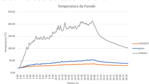
Figura 2. Curvas obtidas na simulação de Incêndio.
