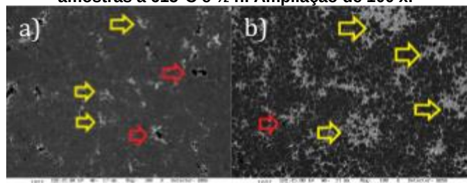
Figura 2: Micrografia: a) amostras à 585^\circ\text{C} e \frac{1}{2}\text{h} ; b) amostras à 615^\circ\text{C} e \frac{1}{2}\text{h} . Ampliação de 100 x.
