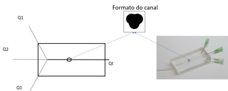
Figura 1: Esquema do microdispositivo que favorece advecção caótica, Q_1 são as correntes aquosas e Q_2 a corrente lipídica, Q_t é a corrente de saída.
