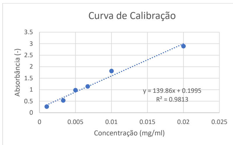
Figura 2: Curva de calibração para a mistura de etanol, lipídio, água e curcumina.
