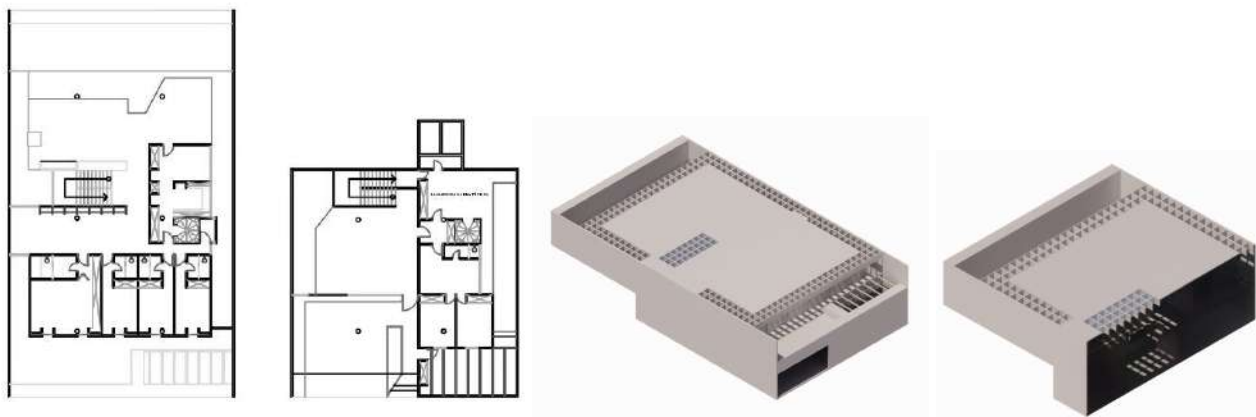
Imagens 10, 11, 12 e 13: Casa Teofilo Orth; Desenhos técnicos das plantas, modelo 3D em perspectiva isométrica e estudo de iluminação com auxílio do corte perspectivado e renderização.
