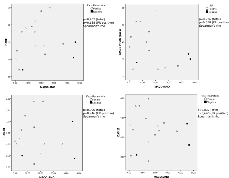
Figura 1 - Intensidade do tabagismo em maço-ano e variáveis contínuas (n=17 no total e n=14 no FR positivo)
