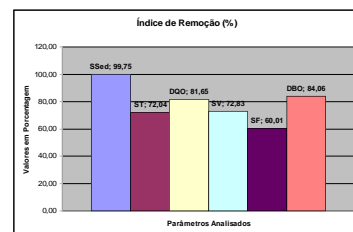
Figura 11 – Porcentagem de Remoção Total
