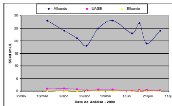
Figura 6 – Evolução Temporal das análises de Sólidos Sedimentáveis (SSed).
