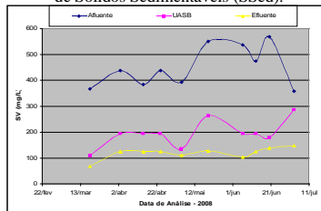
Figura 8 – Evolução Temporal das análises de Sólidos Voláteis (SV).
