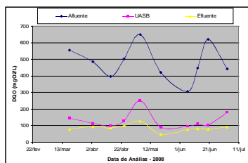
Figura 10 – Evolução Temporal das análises de Demanda Química de Oxigênio (DQO).
