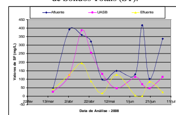
Figura 9 – Evolução Temporal das análises de Sólidos Fixos (SF).
