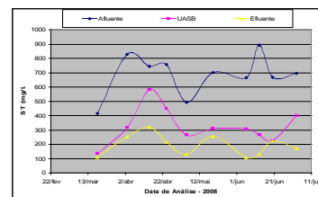
Figura 7 – Evolução Temporal das análises de Sólidos Totais (ST).
